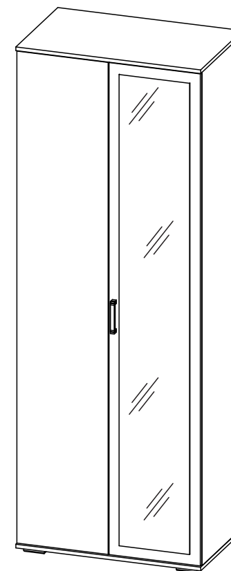
«НЕЛЬСОН» Шкаф ШК04 ↔ 802 ↑ 2197 ↗ 503 «NELSON» Cupboard ShK04
