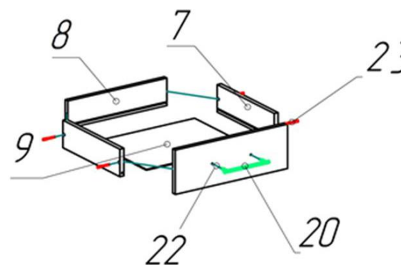
Рисунок 3 – Сборка ящика
