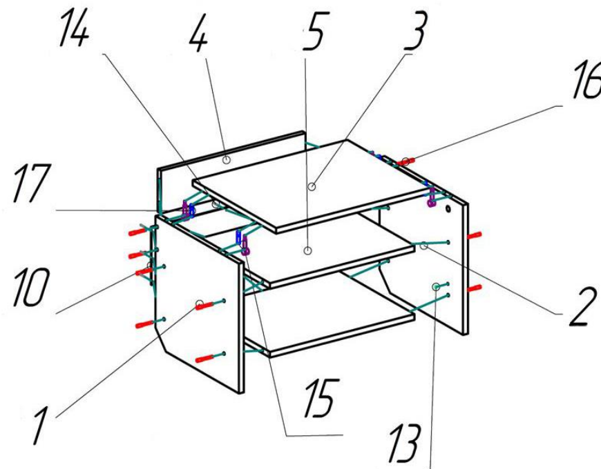
Рисунок 2 – Сборка корпуса
