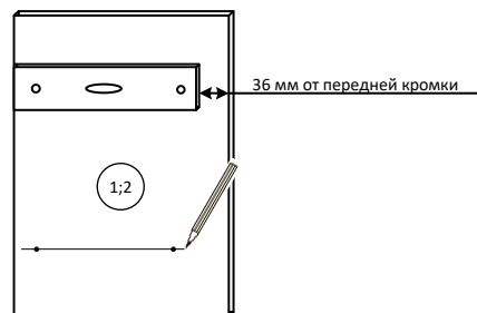
Установка направляющих
