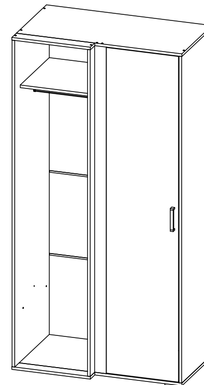
«Денвер» ШКУ Шкаф угловой ↔1000 ↑2020 ↗574 «Denver» SHKU Corner cabinet
