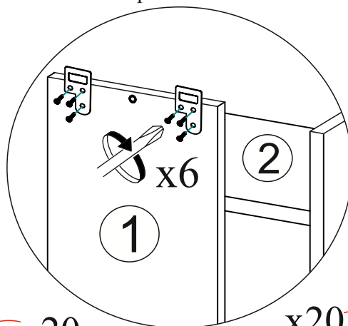
Схема крепления навесов
