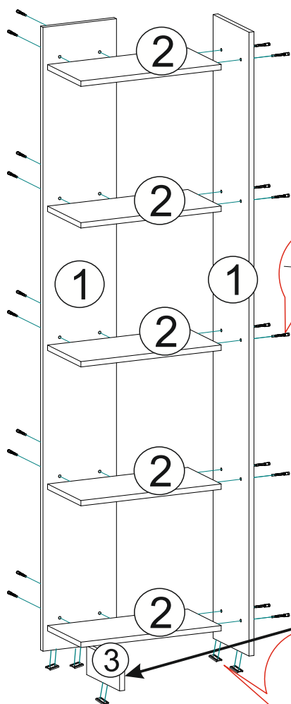
Схема сборки на правую сторону
