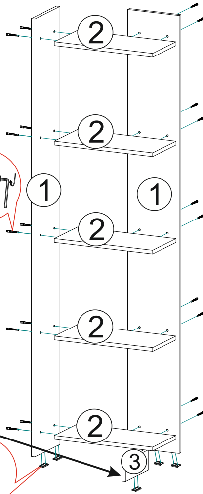
Схема сборки на левую сторону
