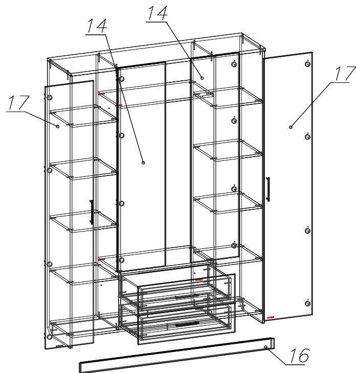
Рисунок 5 – Установка фасадов
