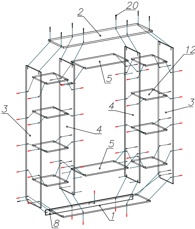
Рисунок 2 – Сборка корпуса
