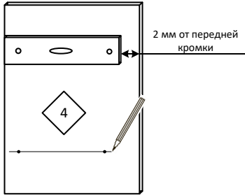
Установка направляющих
