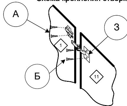
Схема крепления створки
