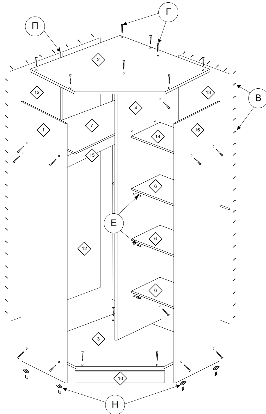
Схема сборки каркаса
