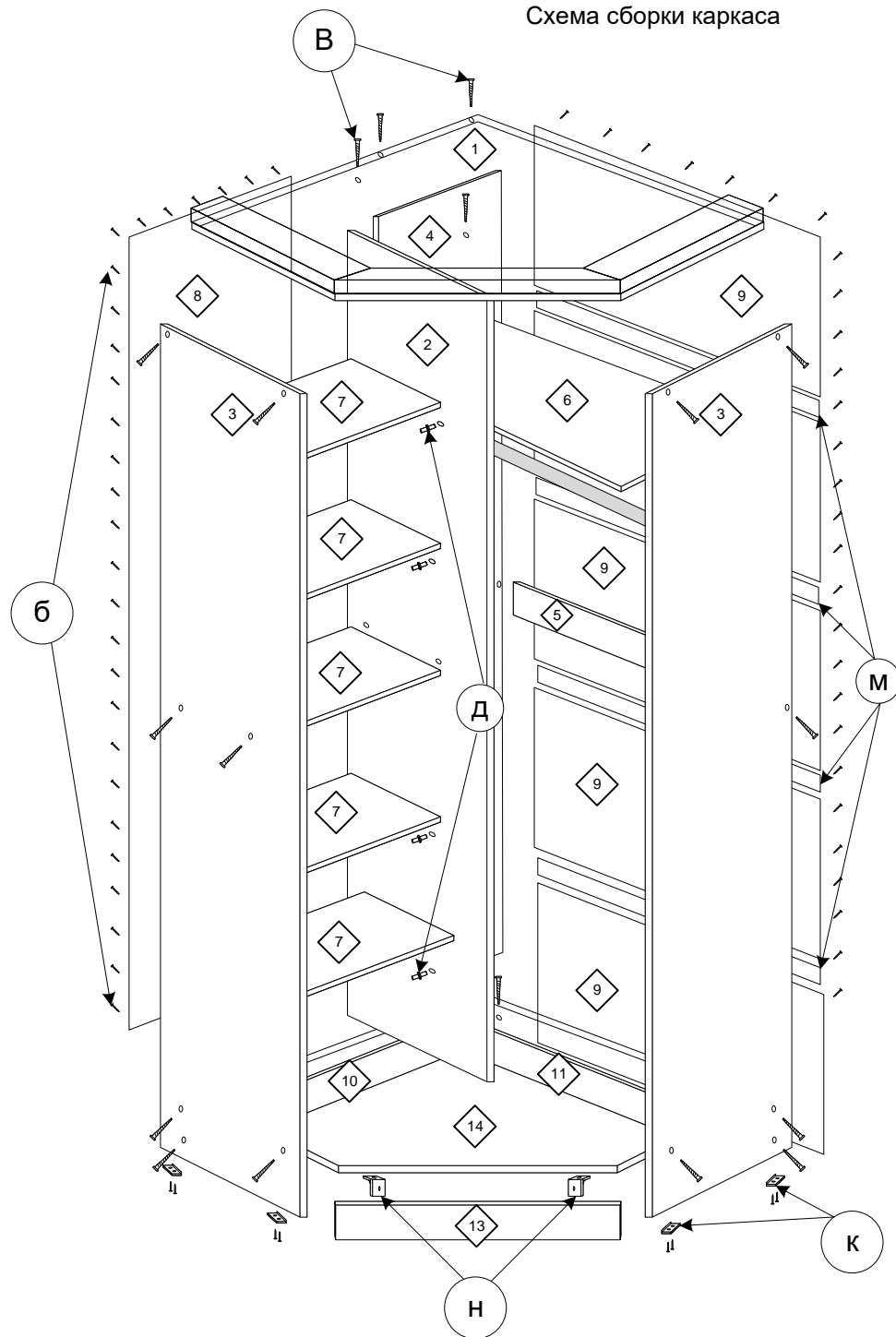
Схема сборки каркаса
